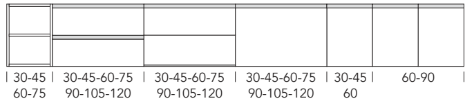
Basi contenitore sospese H.48 P.35/45/50
